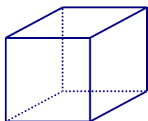
A. Hình lập phương.
