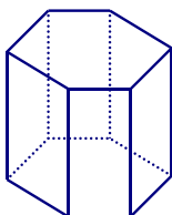
B. Lăng trụ lục giác đều.
