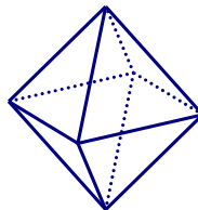
C. Bát diện đều.
