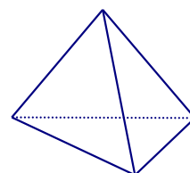
D. Tứ diện đều.
